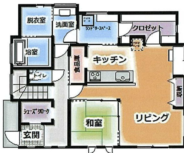
1階
