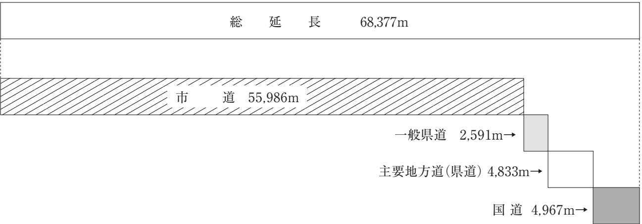
流雪溝敷設状況(令和6年3月31日現在) [8-3 参照]
